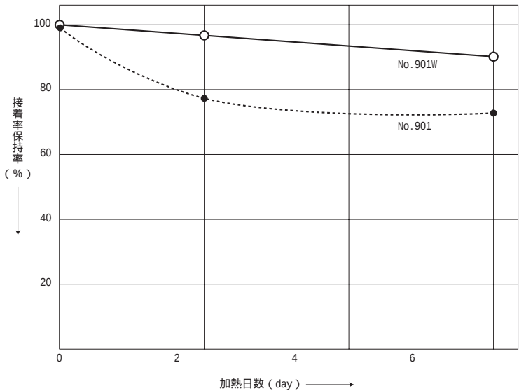
温度180 に加熱したときの加熱日数と接着力変化
