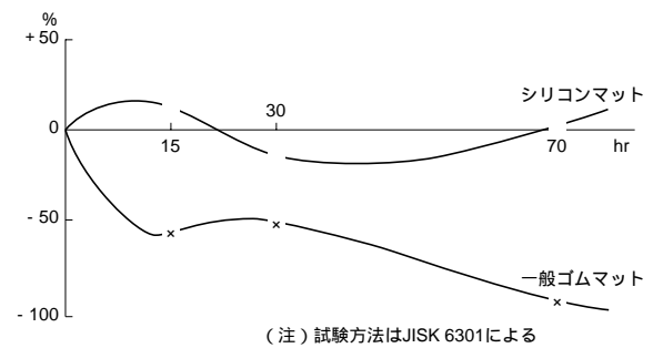
引裂強度 (150 乾熱)
