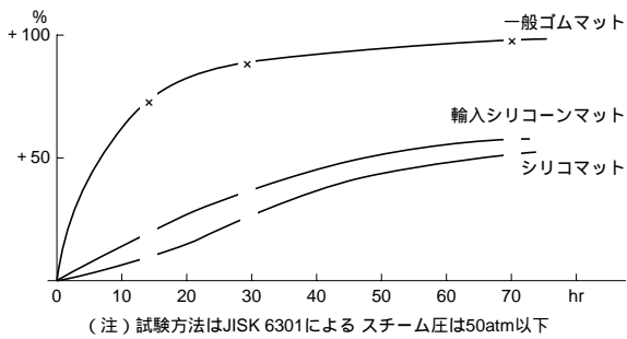
圧縮歪 (100 湿熱)
