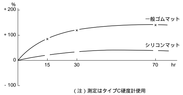
硬度 (150 乾熱)
