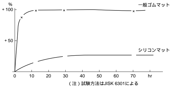
圧縮歪 (150 乾熱)
