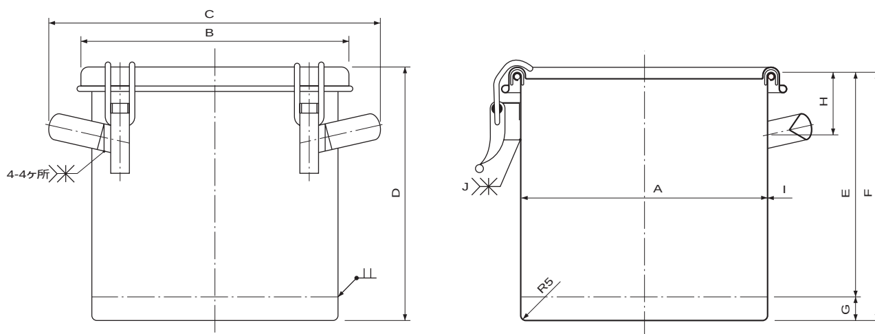
寸法表
