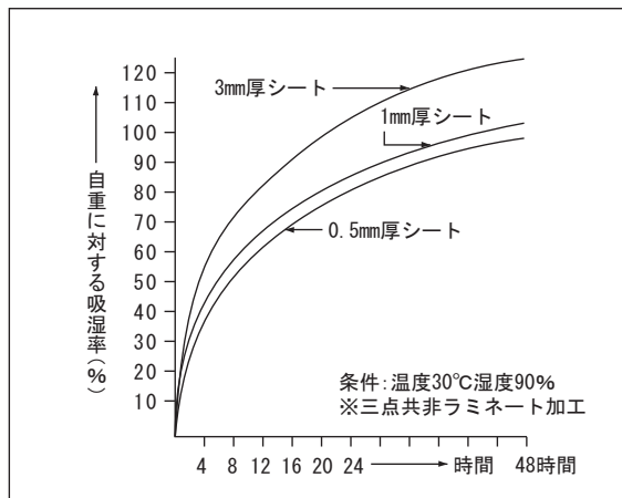
アイディシート状乾燥剤吸湿試験
