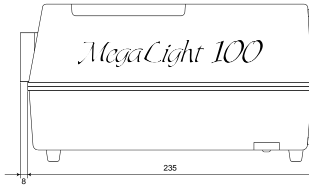
側面
