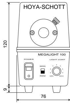
前面
