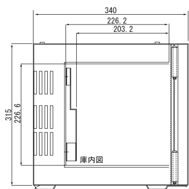
<左側面図>
