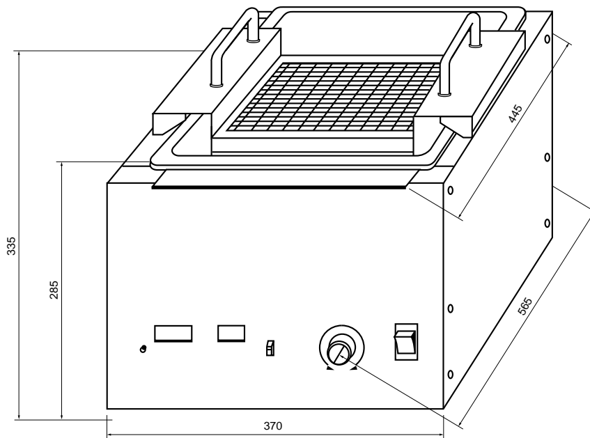
SB-20型の外形寸法図
